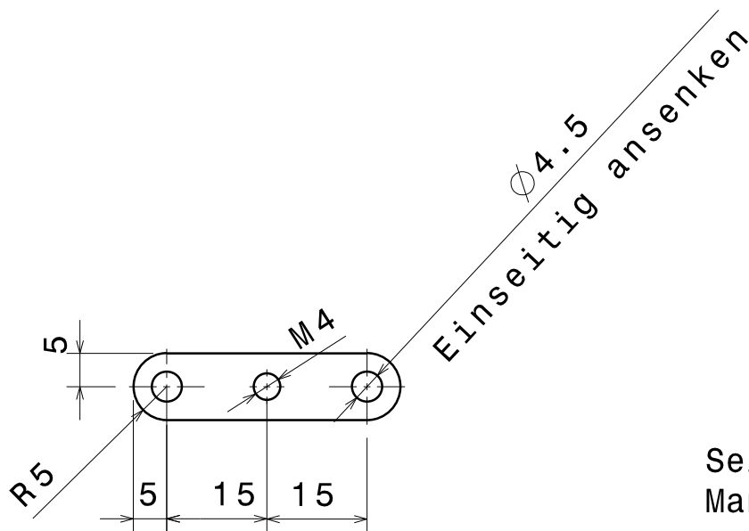
Vorderansicht Maßstab: 1:1
